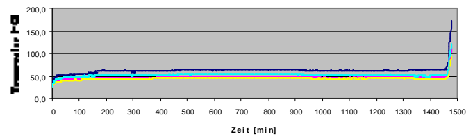
Temperaturverlauf des Dauertests mit anschließender Überlast
